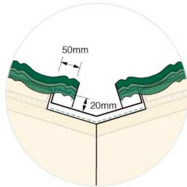
图1.5.3 胶合板层面 在屋面天沟临近处的挂瓦条上,将钉子打入一半,然后将钉子弯曲使其钉帽处能钩住屋面天沟的侧边,以使屋面天沟牢固。不允许在屋面天沟的内部使用钉子。
