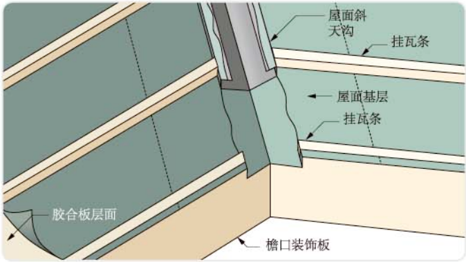
图1.5.3 胶合板层面 在屋面天沟临近处的挂瓦条上,将钉子打入一半,然后将钉子弯曲使其钉帽处能钩住屋面天沟的侧边,以使屋面天沟牢固。不允许在屋面天沟的内部使用钉子。
